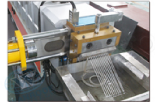
Plastic Strand Die Head 拉条模头
